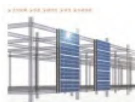
光伏玻璃板装配式墙板
