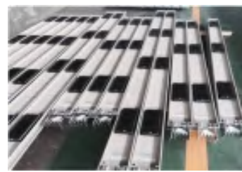
插接式密集母线槽
