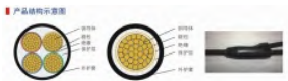
隔离型柔性防火分支电缆
